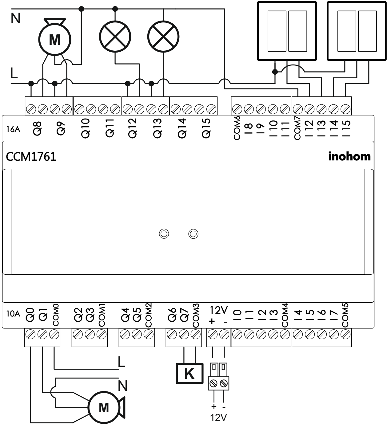
CCM1761 AC Giriş Bağlantı Gösterimi
